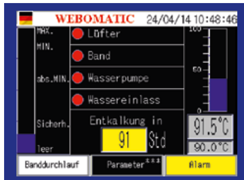
Touchscreen beim Schrumpftunnel STCW.
